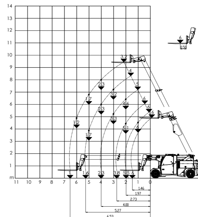
FORCA IDRAULICA DA 6 T
