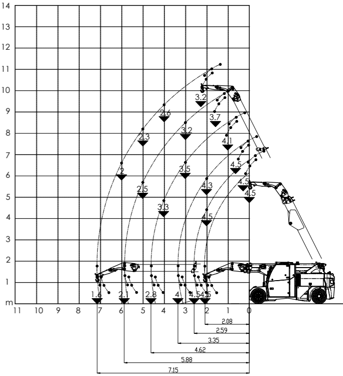
PROLUNGA DA 4,5 t SU JIB MECCANICO POSIZIONE GIU'
