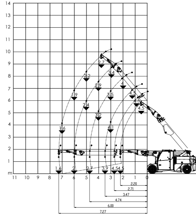
PROLUNGA DA 4,5 t SU JIB MECCANICO POSIZIONE SU
