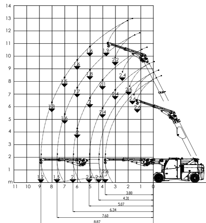
JIB IDRAULICO CORTO POSIZIONE APERTO
