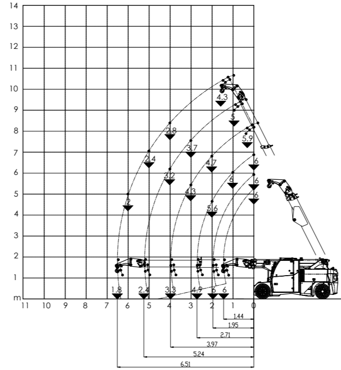
jib MECCANICO 6 T POSIZIONE GIU'
